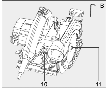
Ill. 24 : fixation de la lame de scie
