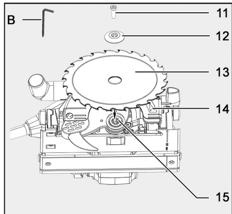
Fig. 41: Cambiar la hoja de sierra
