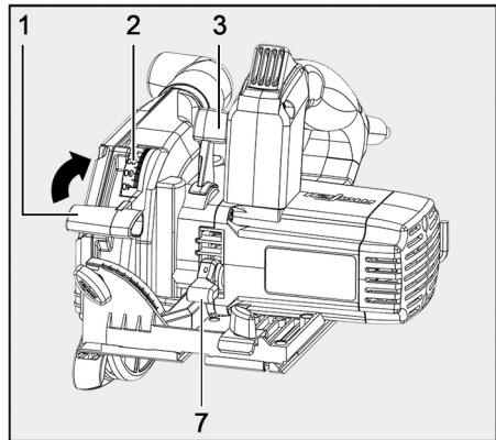
Fig. 48: Realizar el corte de incisión.
