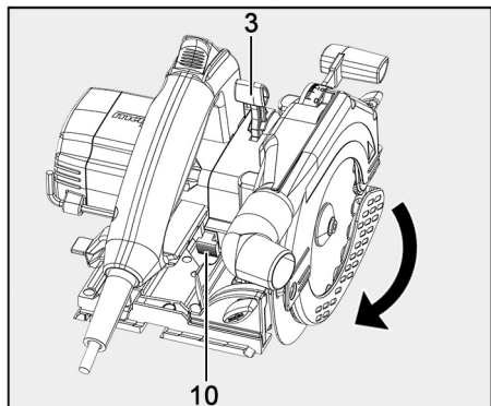
Ill. 21 : blocage de l'arbre de scie
