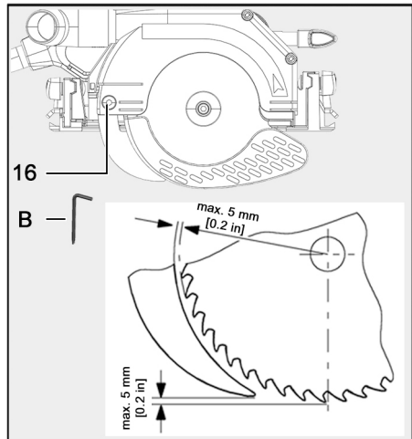
Ill. 25 : Écart entre le couteau diviseur et la lame de scie
