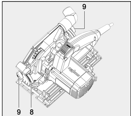
III. 29 : réglage du groupe de sciage pour coupes biaisées
