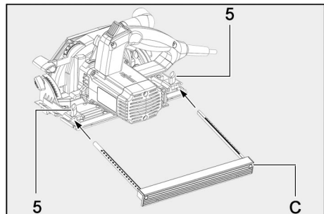
Fig. 53: Colocar el tope paralelo
