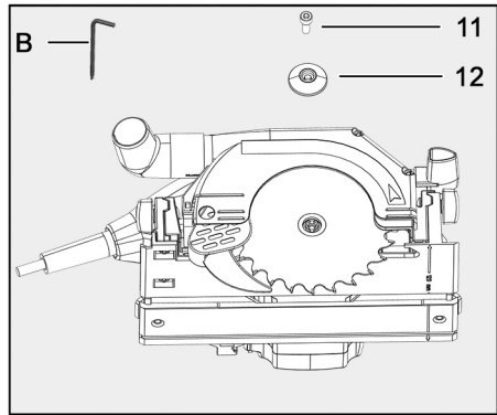
Fig. 40: Retirar la hoja de sierra usada
