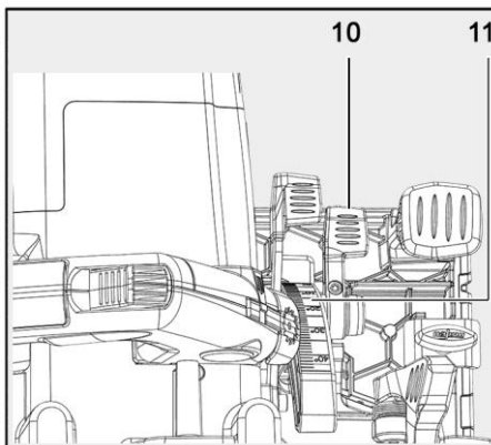
Fig. 70: Ajustar el equipo de sierra para cortes inclinados
