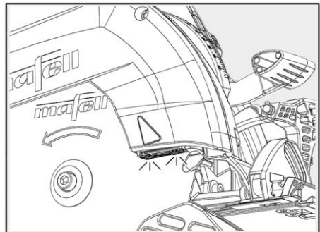
Fig. 66: Módulo de luz de la máquina
