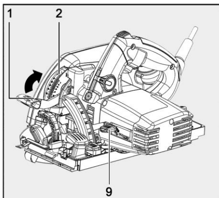
Ill. 43 : réglage de la profondeur de coupe
