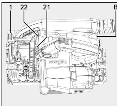
III. 47 : réinitialisation de la profondeur de coupe
