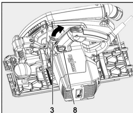
Fig. 59: Bloquear el eje de la sierra
