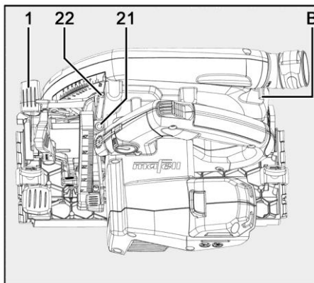
Fig. 72: Preajustar la profundidad de incisión
