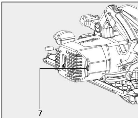
Ill. 41 : réglage de la vitesse de rotation à l'aide de la molette
