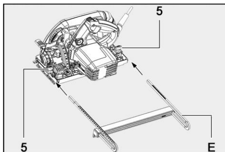
Fig. 77: Colocar el tope inferior
