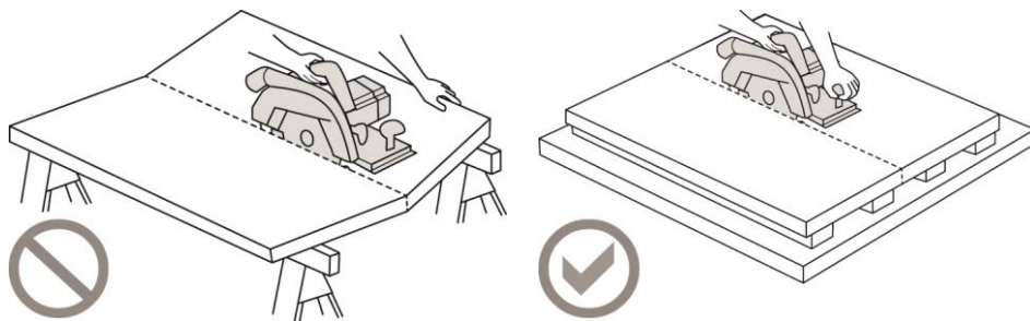
Fig. 57: Apoyo erróneo y apoyo correcto
