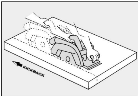
Ill. 30 : rebond de la machine
