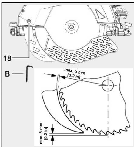
Ill. 38 : Écart entre le couteau diviseur et la lame de scie
