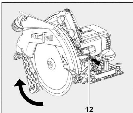
Fig. 60: Abrir la funda protectora
