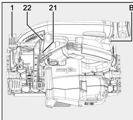
III. 46 : préréglage de la profondeur de plongée
