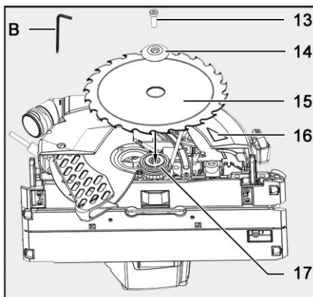
Ill. 36 : remplacement de la lame de scie
