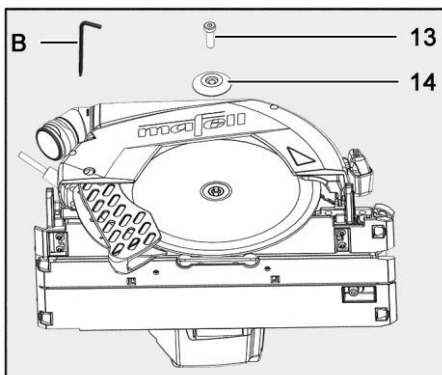
Fig. 61: Retirar la hoja de sierra usada
