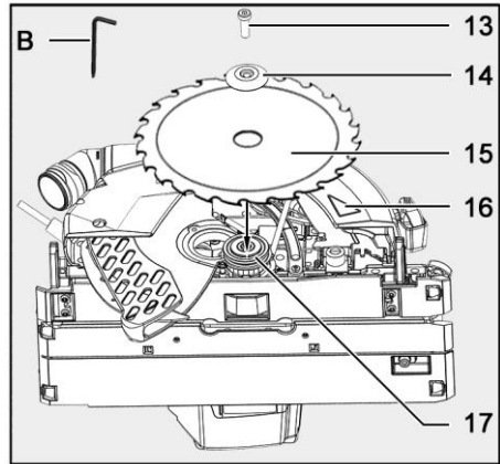
Fig. 62: Cambiar la hoja de sierra
