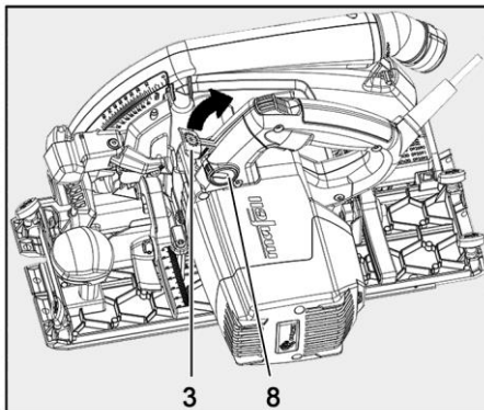
Ill. 33 : blocage de l'arbre de scie
