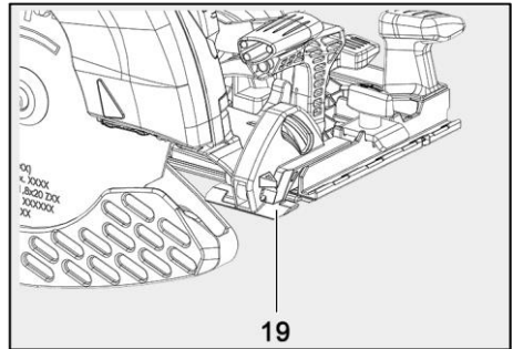
Fig. 74: Canto de trazado
