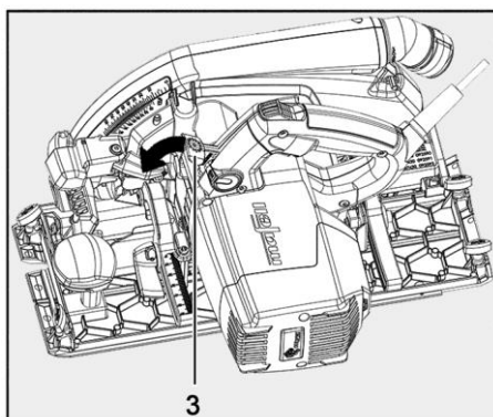
Ill. 37 : déverrouillage du levier de commande
