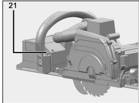
Ill. 49 : rallonge de la coupe longitudinale avec butée de réajustage
