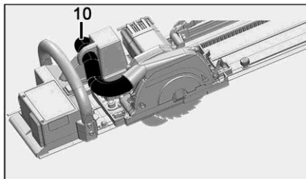
III. 29 : pièce de raccordement entre le groupe de sciage et le canal d'évacuation des copeaux
