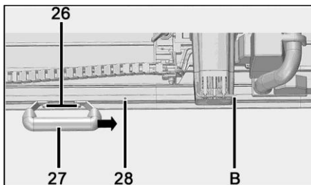
Ill. 52 : déplacement de la poignée étrier pour un transport ergonomique pratique
