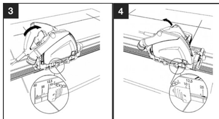
III. 56 : réglage de l'indicateur de position sur la profondeur de coupe
