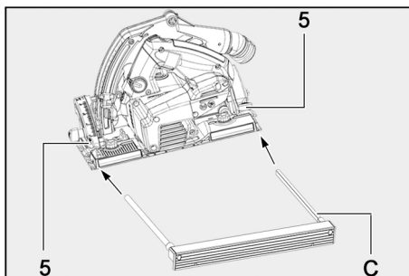
Fig. 76: Colocar el tope paralelo
