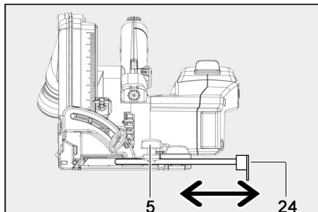
III. 49 : réglage de la largeur de coupe à l'aide du guide parallèle
