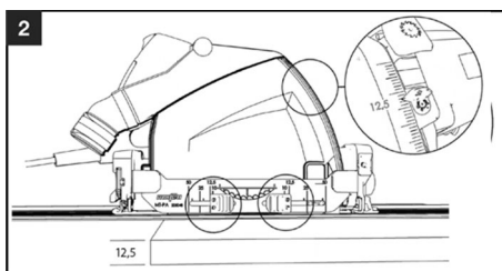
III. 55 : réglage de la profondeur de coupe
