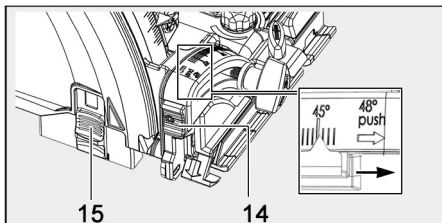
III. 45 : réglage du groupe de sciage sur 48°
