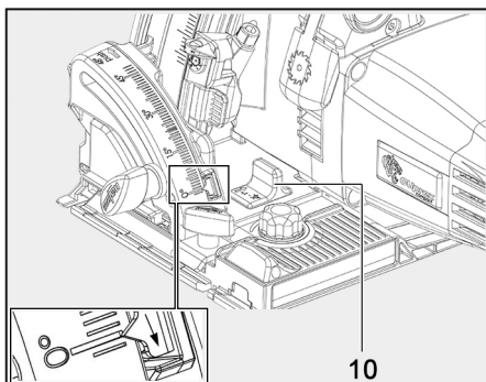
III. 44 : réglage du groupe de sciage sur -1°
