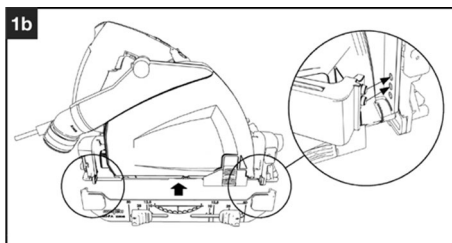
III. 54 : fixation de l'indicateur de position
