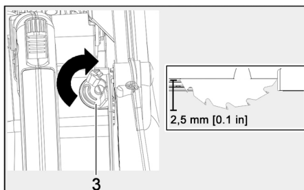
III. 52 : activation de la fonction entaille préalable
