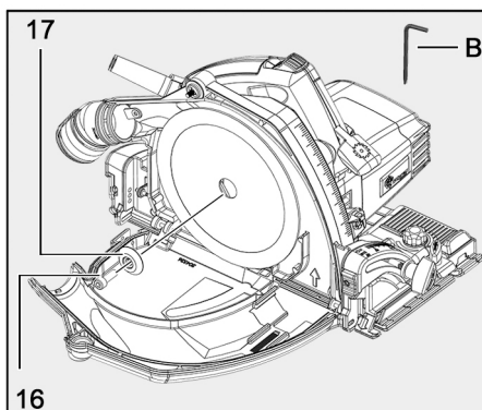
Fig. 63: Retirar la hoja de sierra usada
