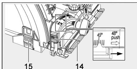
Fig. 73: Ajustar el equipo de sierra a 48°
