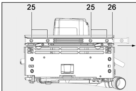
III. 51 : retrait de l'insert pour règles étrangères
