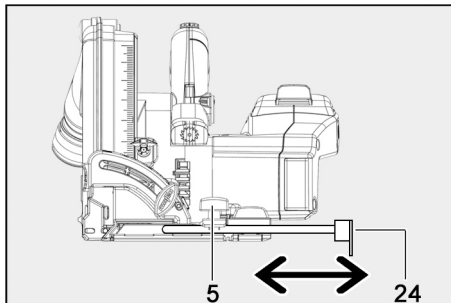
Fig. 77: Ajustar el ancho de corte con el tope paralelo
