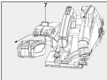
Fig. 60: Desmontar el acumulador
