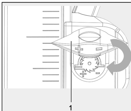
Fig. 69: Posición del indicador profundidad de corte
