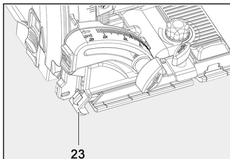
Fig. 19: Tracing edge
