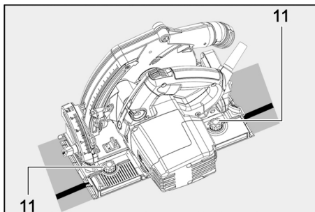
Fig. 78: Ajustar la holgura de la guía
