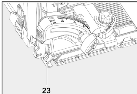
Fig. 75: Canto de trazado
