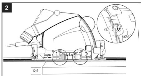
Fig. 83: Ajustar la profundidad de corte
