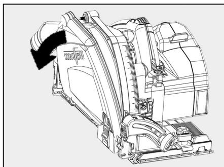
Fig. 62: Abrir la tapa de la funda protectora
