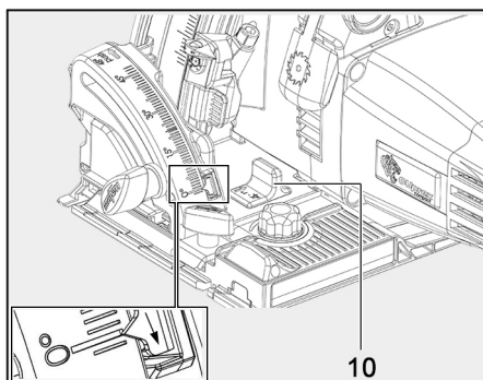
Fig. 72: Ajustar el equipo de sierra a -1°
