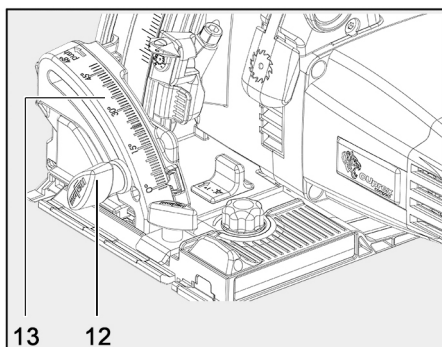
Fig. 71: Ajustar el equipo de sierra para cortes inclinados
