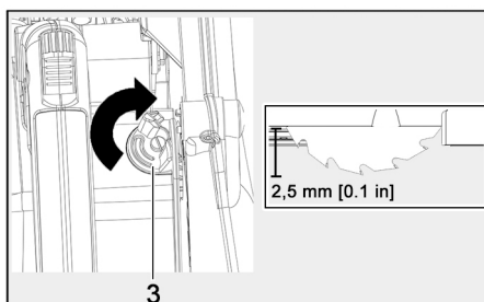
Fig. 80: Activar la función de rasgado
