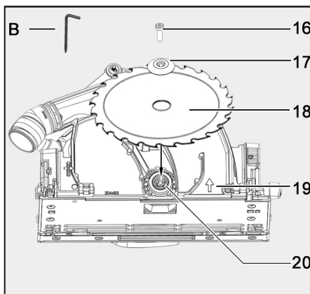
Fig. 64: Cambiar la hoja de sierra
