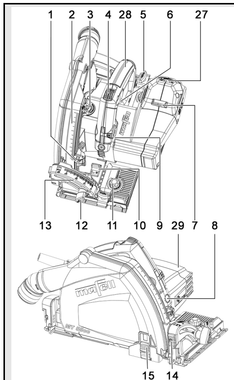
III. 30 : éléments de commande
