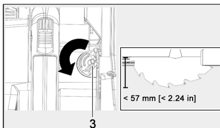
Fig. 81: Desactivar la función de rasgado
