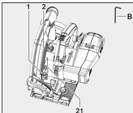
Ill. 42 : réglage de la profondeur de coupe
