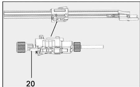
III. 54 : mise en place du rouleau-guide sur la butée latérale
