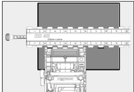
III. 65 : pose de la machine contre le gabarit de perçage
