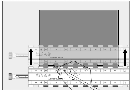
III. 64 : tracé de la position pour gabarit de perçage de tourillons
