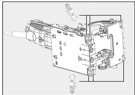
Fig. 92: Puntos de inserción para toques adicionales
