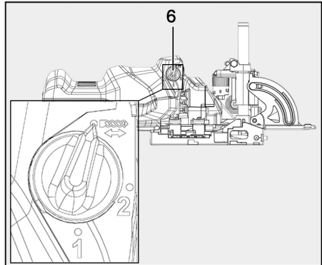
III. 36 : réglage du bouton rotatif sur le pictogramme de changement d'outil
