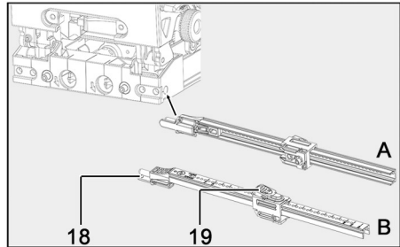
III. 53 : mise en place de la butée latérale sur la machine
