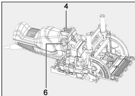
III. 47 : mise en marche/arrêt de la machine
