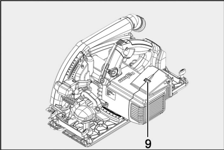
Fig. 61: Ajustar la velocidad con la rosca
