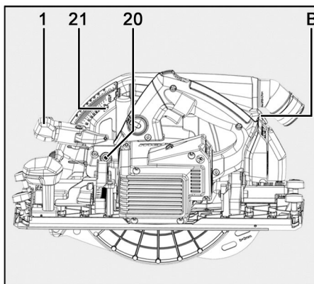
III. 43 : réinitialisation de la profondeur de coupe
