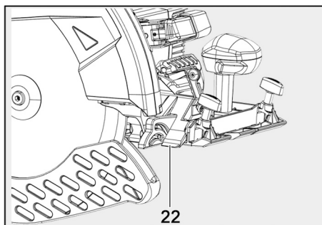
Fig. 20: Tracing edge
