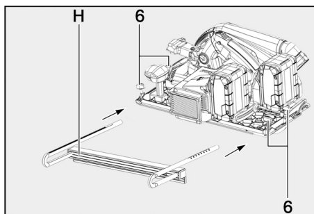
Fig. 71: Colocar el tope inferior
