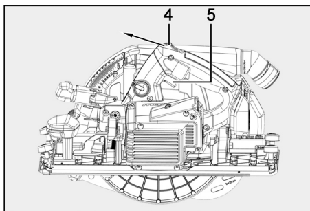
Fig. 59: Conectar la máquina
