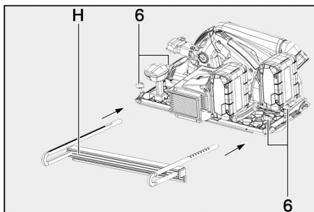
Fig. 23: Installing the roller edge guide
