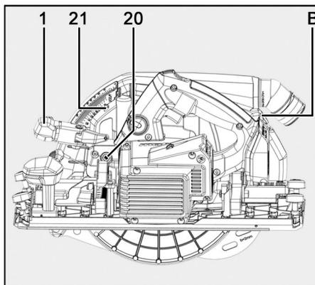
III. 42 : préréglage de la profondeur de plongée
