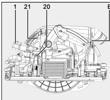
Fig. 66: Preajustar la profundidad de incisión
