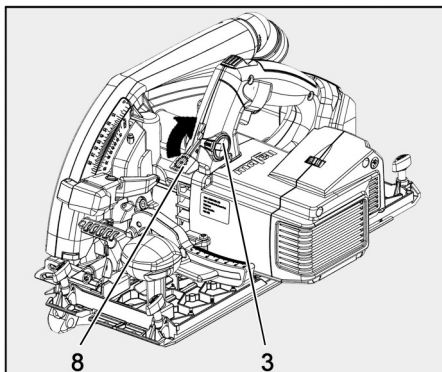
III. 29 : blocage de l'arbre de scie
