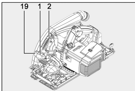
Fig. 63: Ajustar la profundidad de corte
