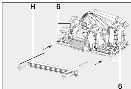
III. 47 : mise en place du rouleau-guide
