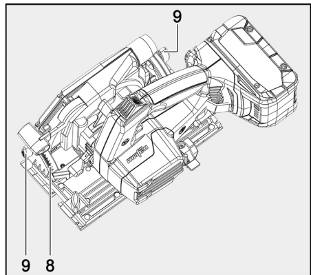
III. 44 : réglage du groupe de sciage pour coupes biaisées
