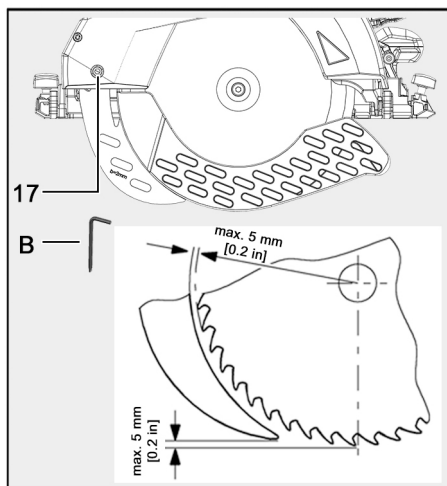
III. 40 : Écart entre le couteau diviseur et la lame de scie
