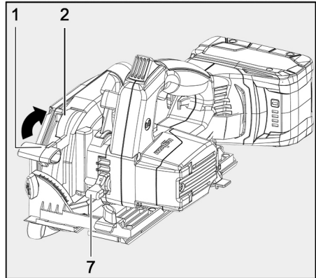
III. 43 : réglage de la profondeur de coupe
