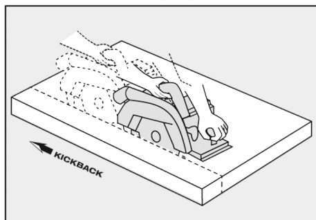
Ill. 31 : rebond de la machine
