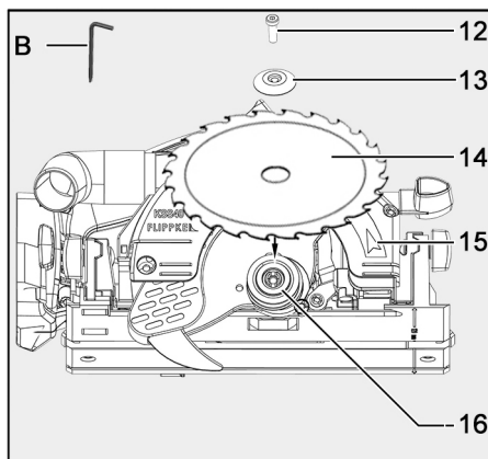
Fig. 65: Cambiar la hoja de sierra
