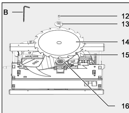
III. 25 : remplacement de la lame de scie
