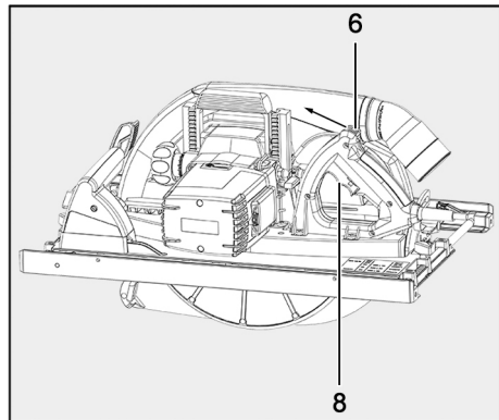
Fig. 44: Conectar la máquina
