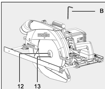
III. 22 : Retirer la vis de bride et la bride de serrage
