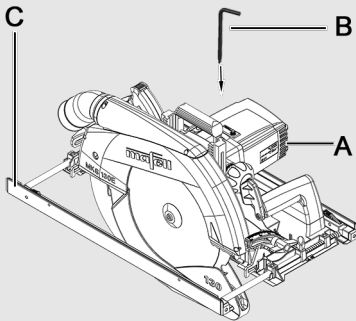
Fig. 35: Contenido MKS 130 Ec
