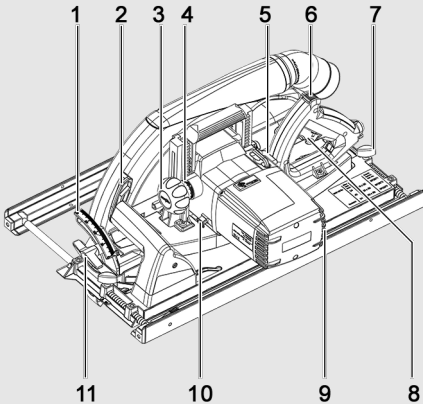
Ill. 19 : éléments de commande MKS 130 Ec
