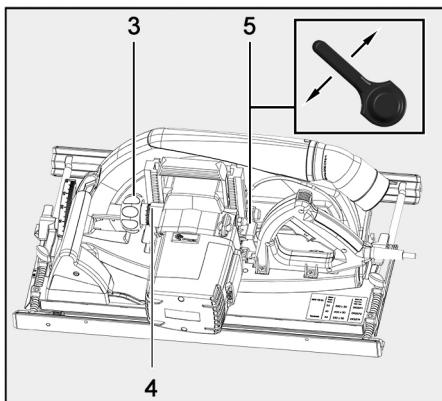
Fig. 47: Ajustar la profundidad de corte
