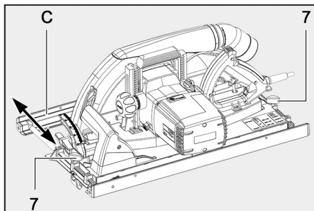
Fig. 50: Ajustar el tope paralelo
