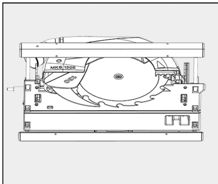
Fig. 41: Retirar la hoja de sierra usada
