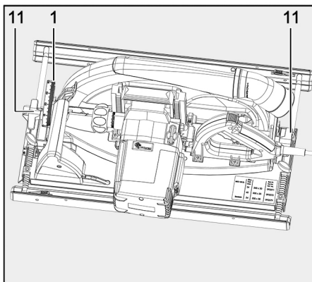
III. 31 : réglage de la scie pour coupes biaisées
