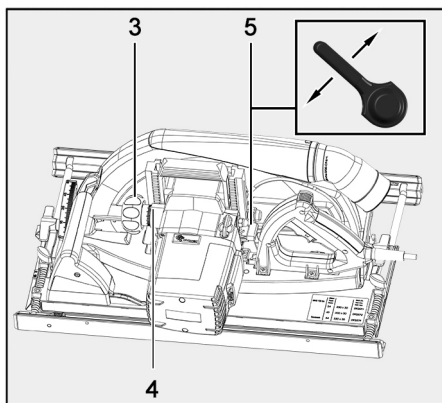
III. 30 : réglage de la profondeur de coupe
