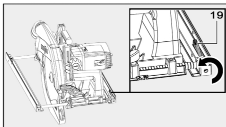
III. 34 : rabattement du côté du guide parallèle.
