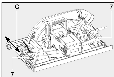
III. 33 : déplacement du guide parallèle
