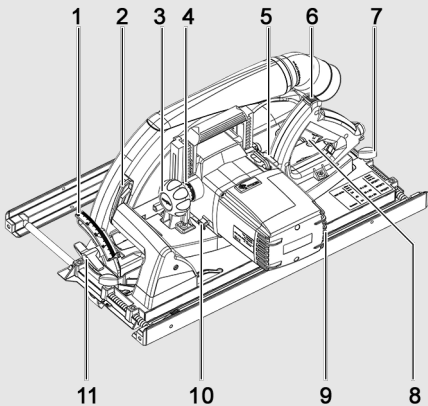
Fig. 36: Mandos MKS 130 Ec
