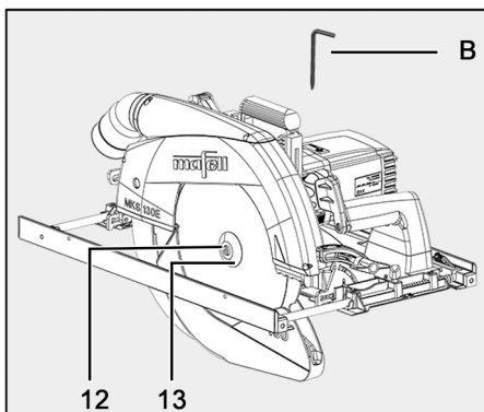
Fig. 39: Retirar el tornillo de brida y la brida de sujeción
