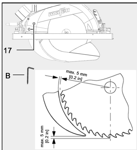
III. 26 : Écart entre le couteau diviseur et la lame de scie
