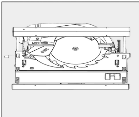
III. 24 : retrait de la lame de scie usée
