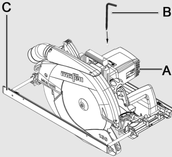
Ill. 18 : équipement standard MKS 130 Ec
