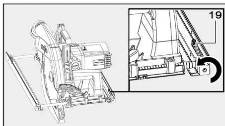
Fig. 51: Abatir el lado del tope paralelo
