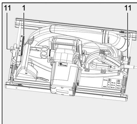
Fig. 48: Ajustar la sierra para cortes inclinados
