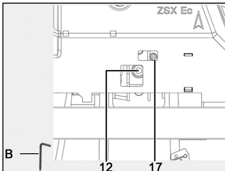
Fig. 96: Ajustar la tensión de la cadena
