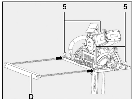
Fig. 107: Colocar el tope paralelo
