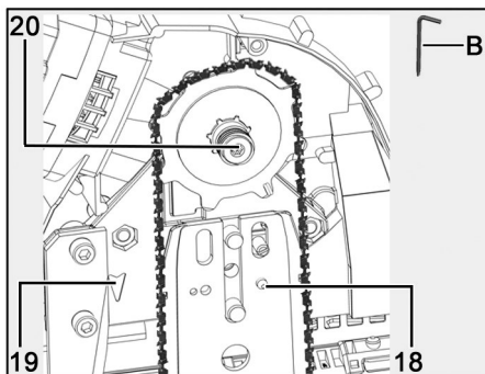
Fig. 88: Colocar la espada de la cadena con una cadena de sierra nueva o recién afilada
