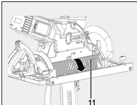
III. 54 : ouverture du clapet de protection
