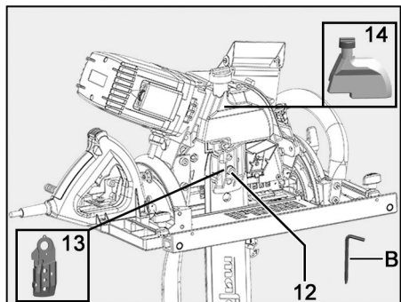
III. 49 : mise en place du couvercle intermédiaire et du réservoir d'huile
