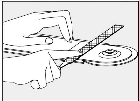
III. 79 : ébavurage du guide-chaîne
