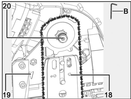
III. 48 : mise en place du guide-chaîne avec chaîne de scie venant d'être affûtée
