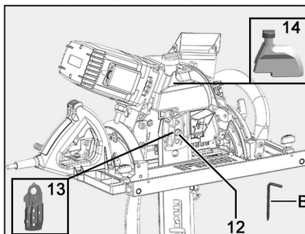
Fig. 89: Colocar la tapa intermedia y el depósito de aceite
