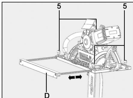
Fig. 108: Ajustar el ancho de corte con el tope paralelo
