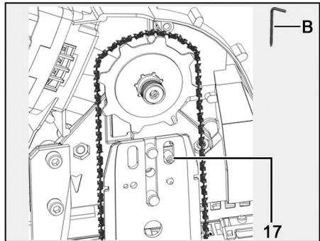
III. 47 : détendre la chaîne et retirer le guide-chaîne y compris la chaîne de scie
