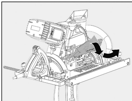
III. 44 : retrait du couvercle
