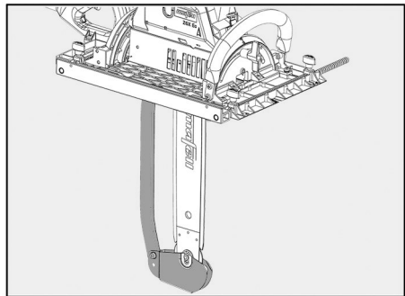
III. 75 : couteau diviseur et protection du renvoi inférieur de chaîne
