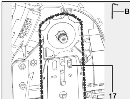
Fig. 87: Soltar la tensión de la cadena y quitar la espada de cadena junto con la cadena de sierra
