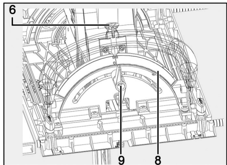
III. 71 : réglage pour coupe d'angle
