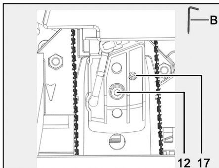
III. 50 : serrage de la tension de chaîne
