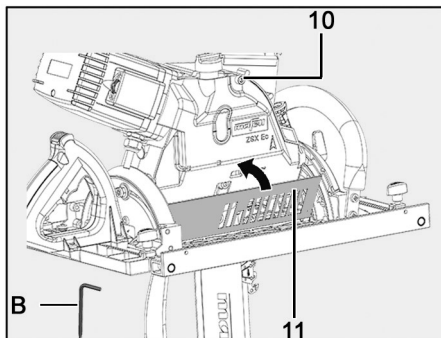
Fig. 93: Cerrar la tapa protectora
