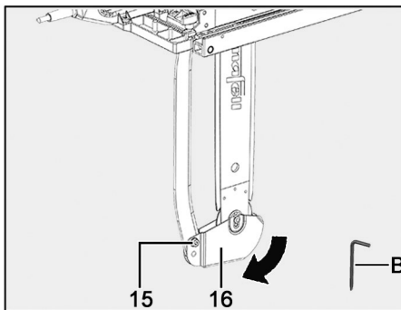
III. 55 : ouverture de la tôle de protection sur le guide-chaîne
