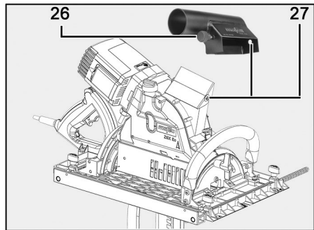
Fig. 117: Colocar el adaptador de absorción
