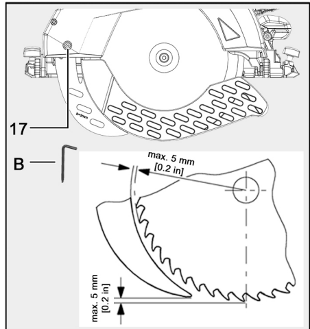
III. 32 : Écart entre le couteau diviseur et la lame de scie
