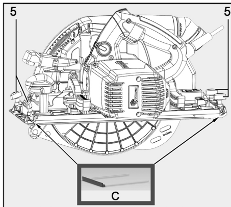
Fig. 66: Colocar el tope paralelo
