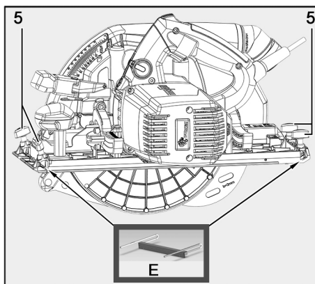
Fig. 68: Colocar el tope inferior
