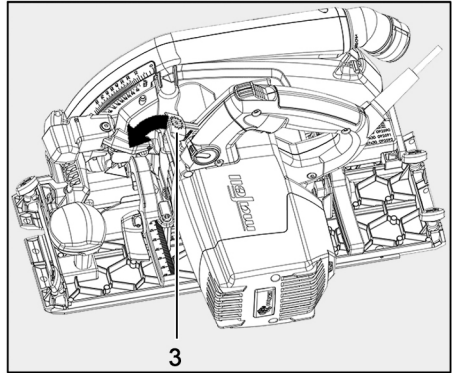
III. 31 : fermeture du capot protecteur
