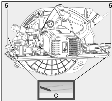
III. 43 : mise en place du guide parallèle
