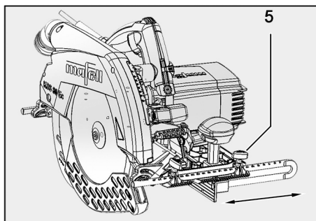
Fig. 69: Ajustar el ancho de corte con el tope inferior
