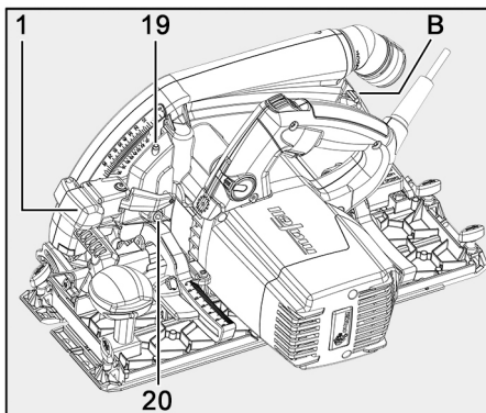
Fig. 63: Preajustar la profundidad de incisión
