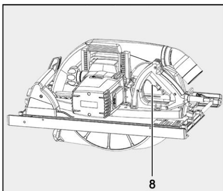
Ill. 35 : arrêter la machine
