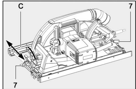
Fig. 59: Ajustar el tope paralelo
