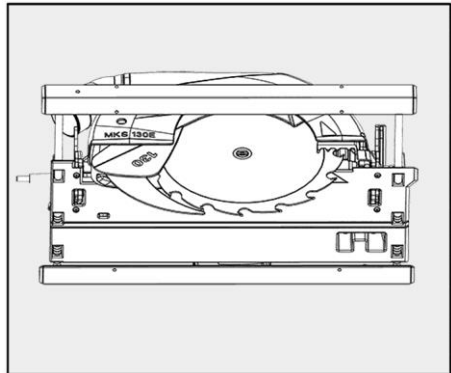
Fig. 50: Retirar la hoja de sierra usada
