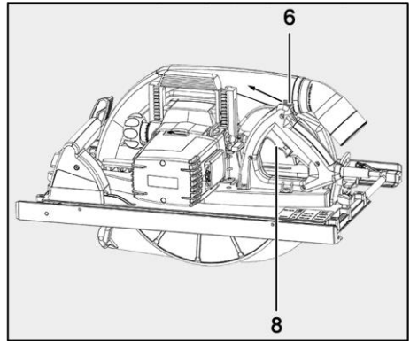
Fig. 53: Conectar la máquina
