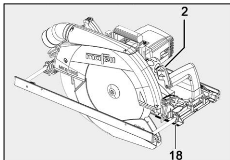
Ill. 38 : bord de traçage
