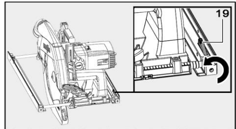
Fig. 60: Abatir el lado del tope paralelo
