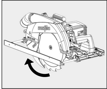
Fig. 49: Abrir la funda protectora
