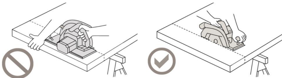
Ill. 23 : sciage de manière incorrecte et incorrecte
