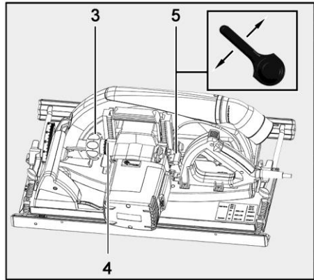
Fig. 56: Ajustar la profundidad de corte
