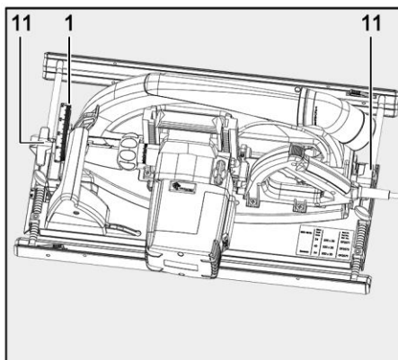
Ill. 37 : réglage de la scie pour coupes biaisées
