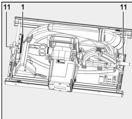
Fig. 57: Ajustar la sierra para cortes inclinados
