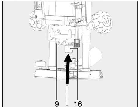
III. 32 : serrage de l'outil de fraisage
