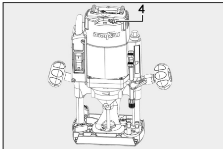
III. 36 : réglage de la vitesse de rotation
