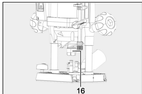
III. 29 : remplacement de la pince de serrage
