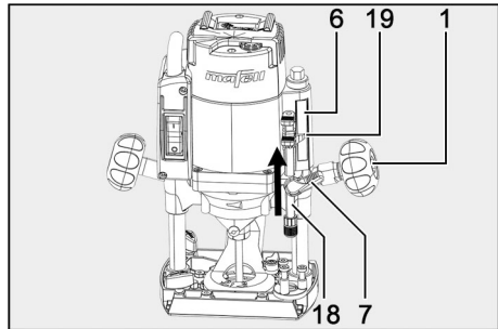
III. 40 : réglage de la butée de profondeur
