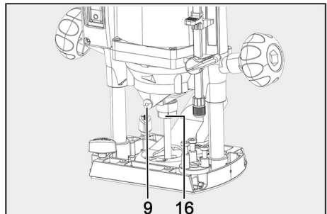
III. 33 : desserrage de l'outil de fraisage
