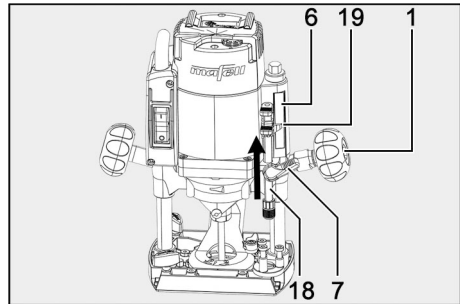
Fig. 63: Ajustar el tope de profundidad
