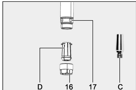
III. 28 : pince de serrage, écrou-raccord, adaptateur et broche de fraisage
