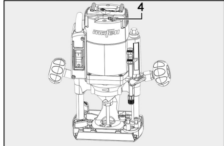
Fig. 59: Ajuste de la velocidad de marcha
