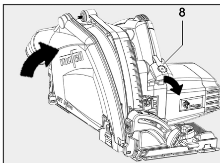
III. 41 : fermeture du capot protecteur
