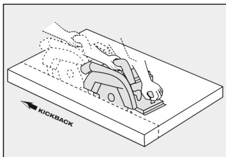
III. 34 : rebond de la machine
