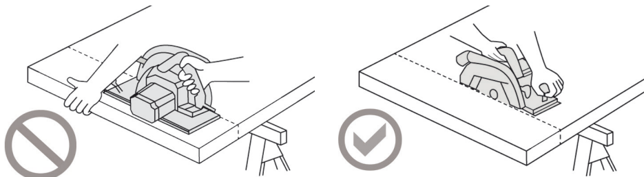
III. 33 : sciage de manière incorrecte et incorrecte
