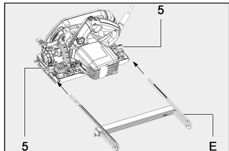
Fig. 19: Installing the roller edge guide
