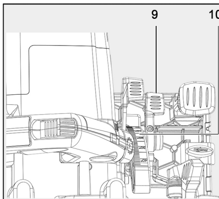
III. 34 : réglage du groupe de sciage pour coupes biaisées
