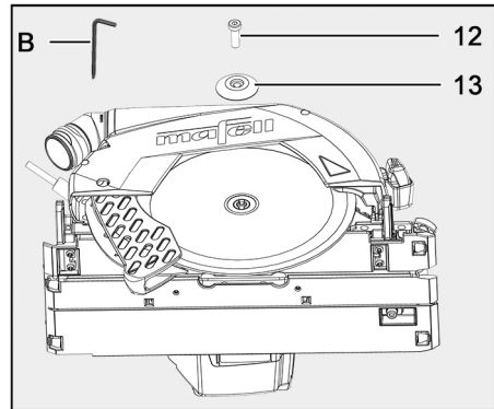
Fig. 46: Retirar la hoja de sierra usada
