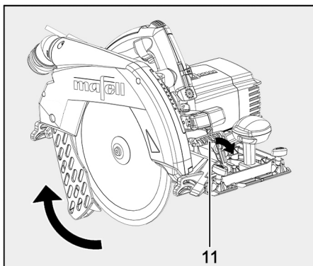
III. 25 : ouverture du capot protecteur
