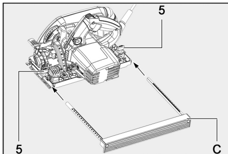
III. 37 : mise en place du guide parallèle
