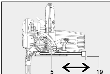
III. 38 : réglage de la largeur de coupe à l'aide du guide parallèle
