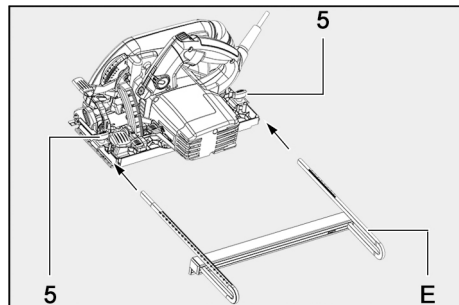
Fig. 59: Colocar el tope inferior
