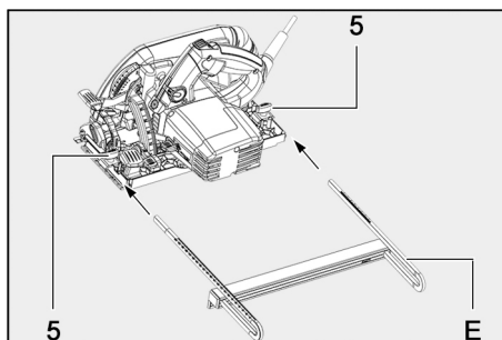
III. 39 : mise en place du rouleau-guide
