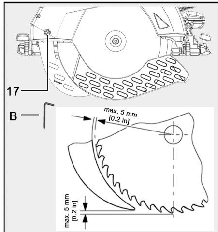
III. 29 : Écart entre le couteau diviseur et la lame de scie
