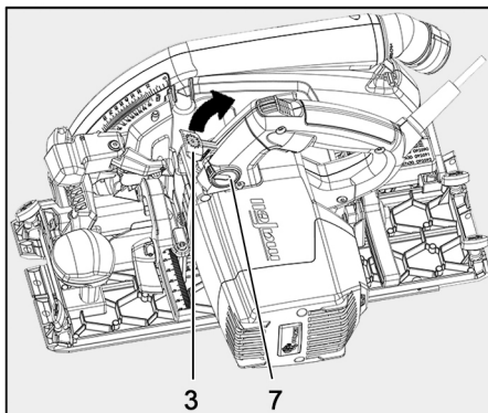
III. 24 : blocage de l'arbre de scie
