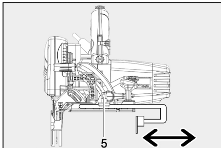
III. 40 : réglage de la largeur de coupe à l'aide du rouleau-guide
