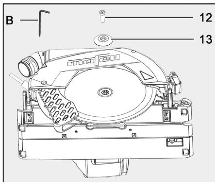
III. 26 : retrait de la lame de scie usée
