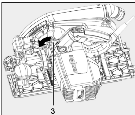
Fig. 48: Desbloquear la palanca de conmutación
