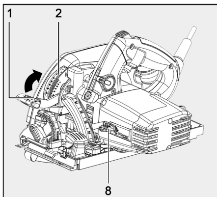
Fig. 53: Ajustar la profundidad de corte
