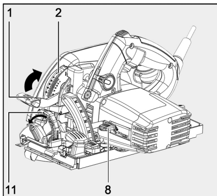
Fig. 55: Realizar el corte de incisión.
