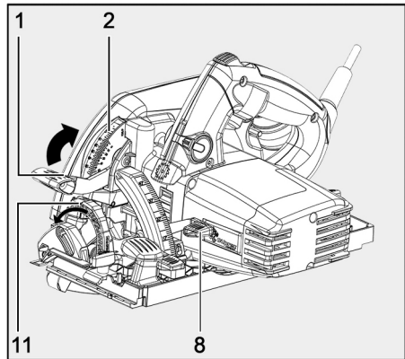
III. 35 : coupe en plongée
