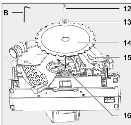
III. 27 : remplacement de la lame de scie
