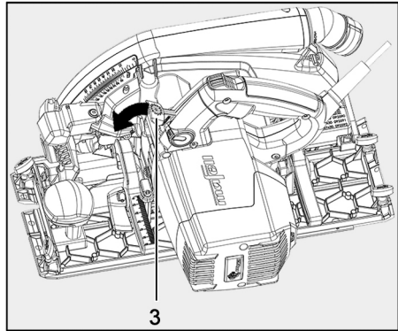
III. 28 : déverrouillage du levier de commande
