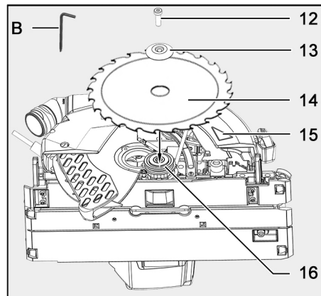
Fig. 47: Cambiar la hoja de sierra
