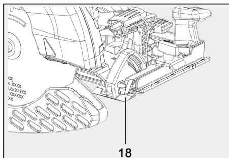
Ill. 36 : bord de traçage
