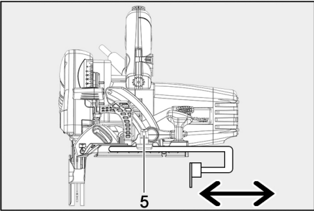
Fig. 60: Ajustar el ancho de corte con el tope inferior
