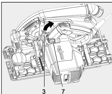
Fig. 44: Bloquear el eje de la sierra
