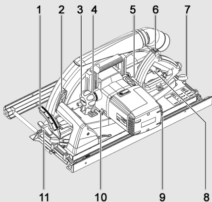
III. 19 : éléments de commande
