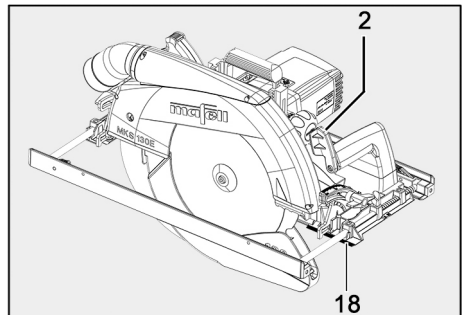
III. 32 : bord de traçage
