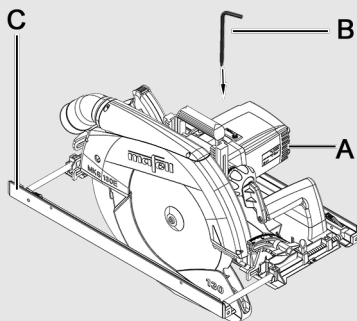
III. 18 : équipement standard
