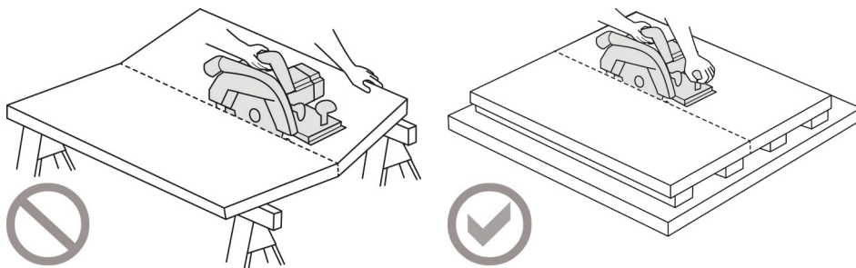
III. 25 : appui incorrect et correct
