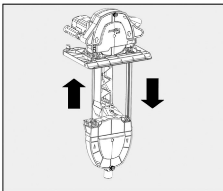
Fig. 74: Dirección de giro del rodillo de sierra sin fin
