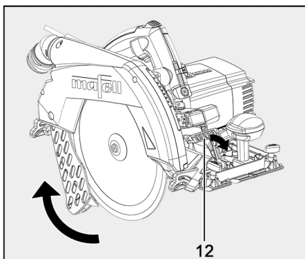
III. 28 : ouverture du capot protecteur
