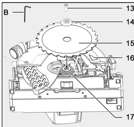
Fig. 53: Cambiar la hoja de sierra
