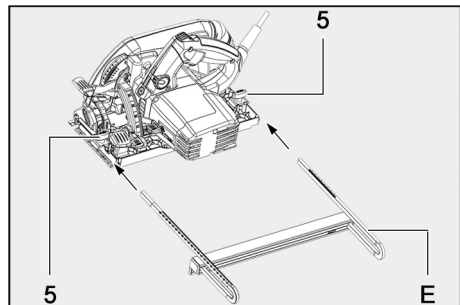
III. 45 : mise en place du rouleau-guide
