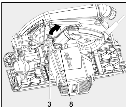
Fig. 50: Bloquear el eje de la sierra
