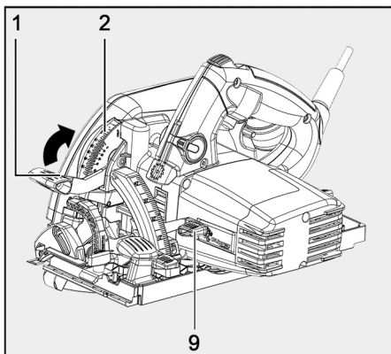
Fig. 60: Ajustar la profundidad de corte
