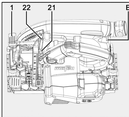
Fig. 64: Restablecer la profundidad de corte
