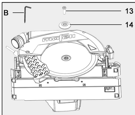
Fig. 52: Retirar la hoja de sierra usada
