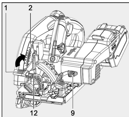
Ill. 45 : coupe en plongée
