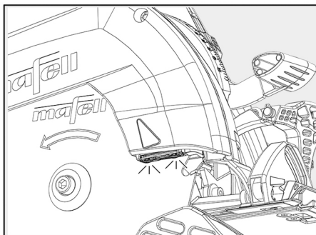
Ill. 41 : module d'éclairage sur la machine
