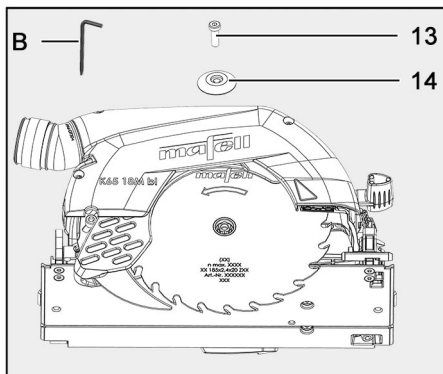
III. 36 : retrait de la lame de scie usée
