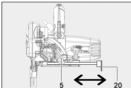
Ill. 50 : réglage de la largeur de coupe à l'aide du guide parallèle
