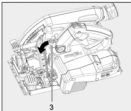
III. 38 : déverrouillage du levier de commande
