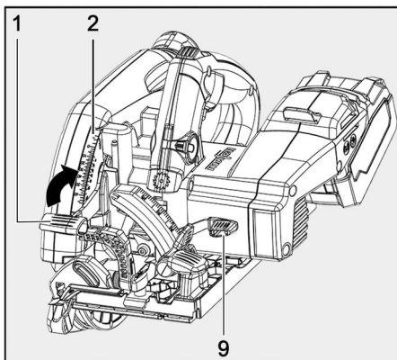
III. 43 : réglage de la profondeur de coupe
