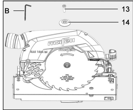
Fig. 62: Retirar la hoja de sierra usada
