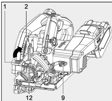
Fig. 71: Realizar el corte de incisión.
