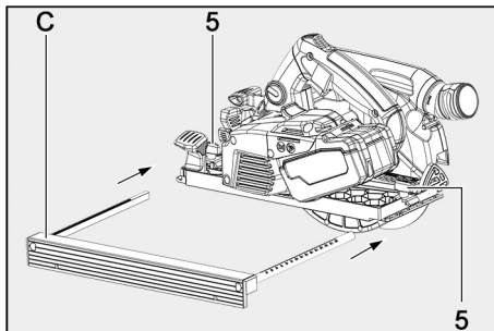
Ill. 49 : mise en place du guide parallèle
