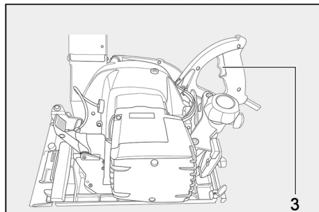
III. 38 : arrêter la machine
