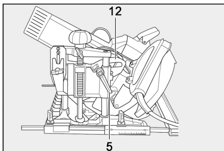
III. 55 : réglage de la fraise pour travaux d'aplanissement
