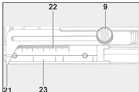
III. 42 : détail de la graduation de traçage
