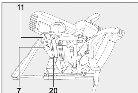
III. 44 : réglage de l'indicateur de profondeur de réglage
