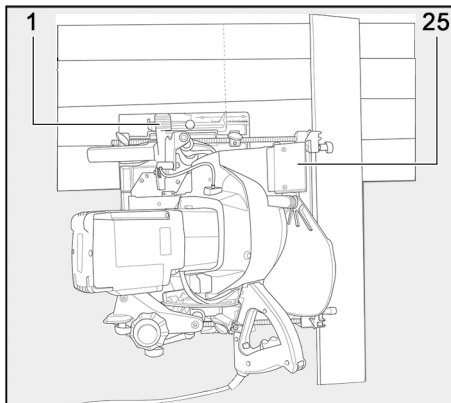
III. 51 : usinage avec le rail de guidage
