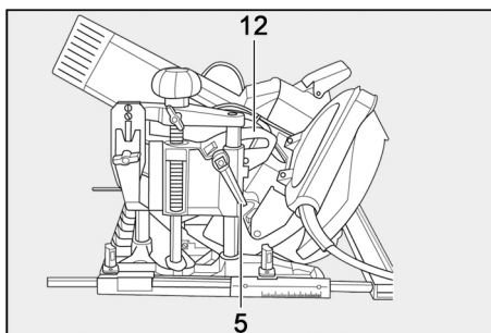
III. 43 : réglage de la fraise pour des travaux d'inclinaison et d'encoche
