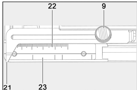
Fig. 70: Imagen detallada escala de marcaje
