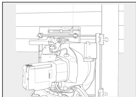
III. 50 : contrôler de la position du traçage à l'aide des graduations de traçage.
