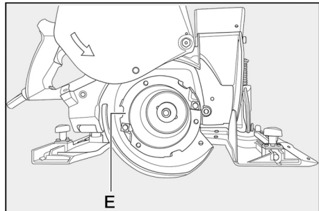
Fig. 62: Quitar el cabezal de fresar
