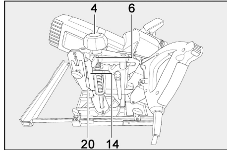
III. 45 : réglage de la profondeur de fraisage
