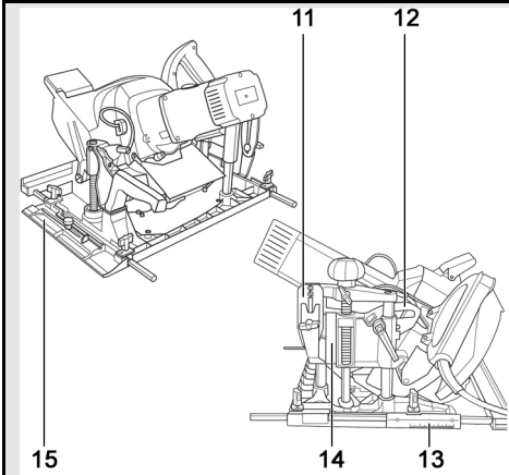
Ill. 31 : graduations sur la ZK 115 Ec
