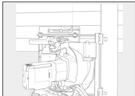
Fig. 78: Comprobar la posición de la línea de trazado mediante las escalas de la línea de trazado
