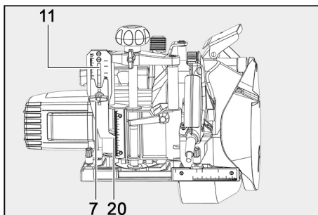
III. 56 : réglage de la profondeur de fraisage sur la machine
