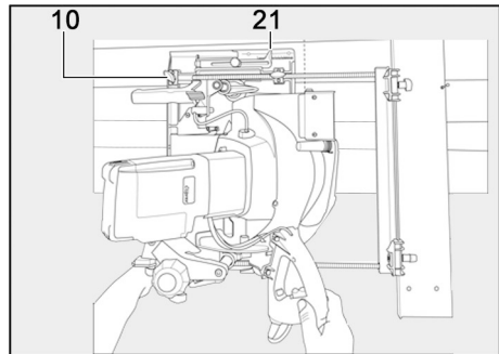
Fig. 77: Posicionar la máquina con respecto a la línea de trazado
