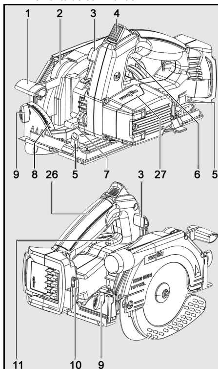
III. 26 : éléments de commande à l'avant et arrière
