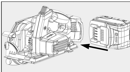
III. 27 : mise en place du bloc batterie dans la machine
