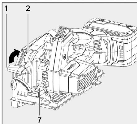
Fig. 61: Ajustar la profundidad de corte
