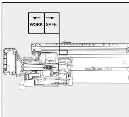
Fig. 72: Realizar corte en inglete con dispositivo guía.
