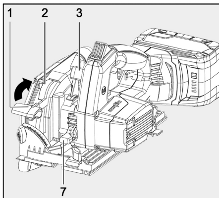
Fig. 63: Realizar el corte de incisión.
