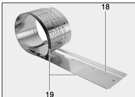
Fig. 65: Recortar la protección contra virutas
