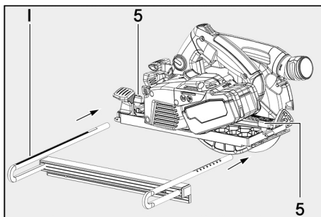
Fig. 65: Colocar el tope inferior
