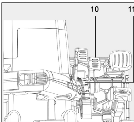
Fig. 60: Ajustar el equipo de sierra para cortes inclinados
