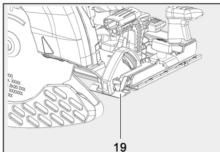
Fig. 18: Tracing edge
