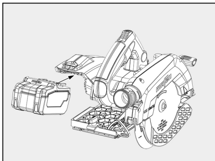
III. 25 : mise en place du bloc batterie dans la machine
