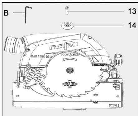
Fig. 51: Retirar la hoja de sierra usada
