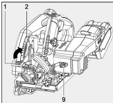
Fig. 59: Ajustar la profundidad de corte
