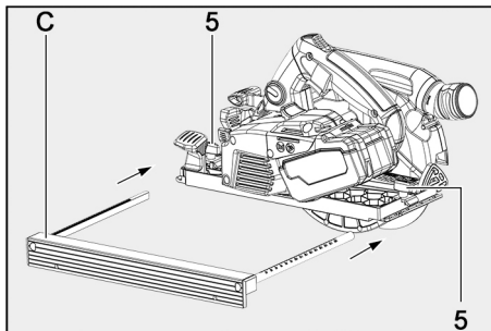
Fig. 63: Colocar el tope paralelo
