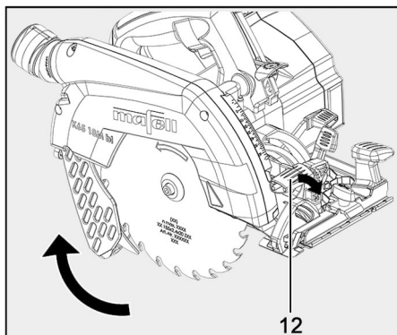
Fig. 50: Abrir la funda protectora
