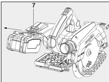
Fig. 48: Desmontar el acumulador
