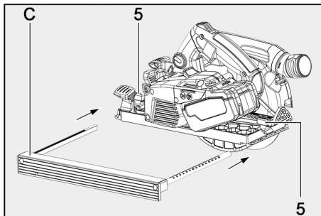
III. 41 : mise en place du guide parallèle
