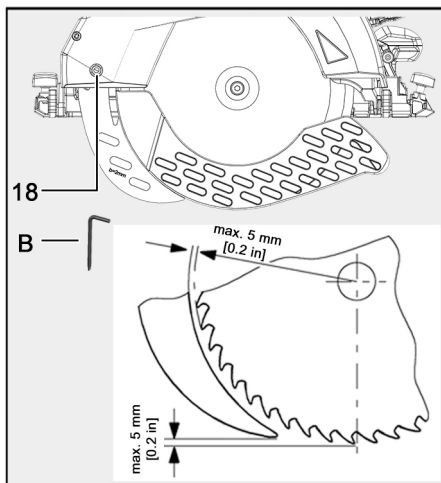
Ill. 32 : écart entre le couteau diviseur et la lame de scie
