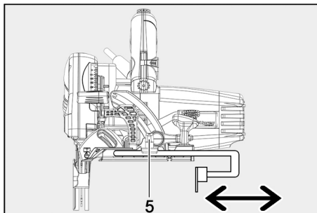
Fig. 66: Ajustar el ancho de corte con el tope inferior
