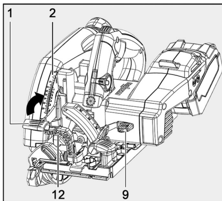
Fig. 61: Realizar el corte de incisión.
