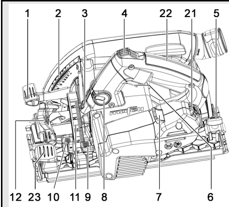
III. 24 : éléments de commande
