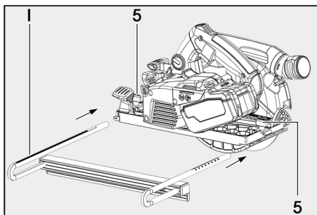
III. 43 : mise en place du rouleau-guide
