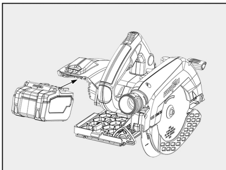
Fig. 47: Colocar la batería en la máquina
