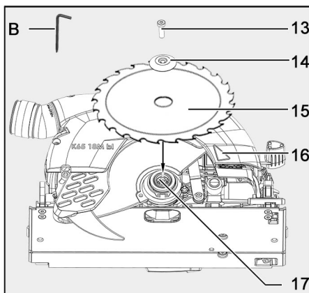
Fig. 52: Cambiar la hoja de sierra
