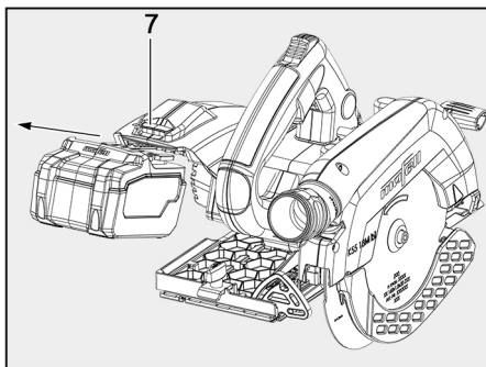
III. 26 : retrait du bloc batterie
