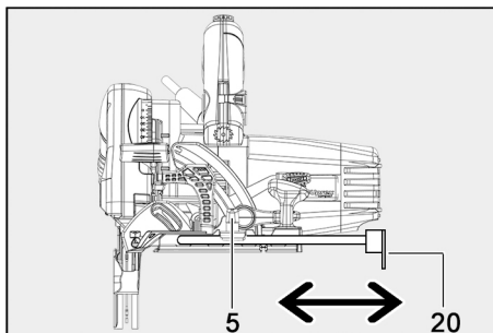
Fig. 64: Ajustar el ancho de corte con el tope paralelo
