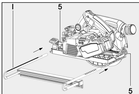
Fig. 21: Installing the roller edge guide
