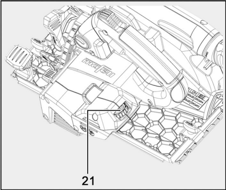
Ill. 35 : réglage de la vitesse de rotation à l'aide de la molette
